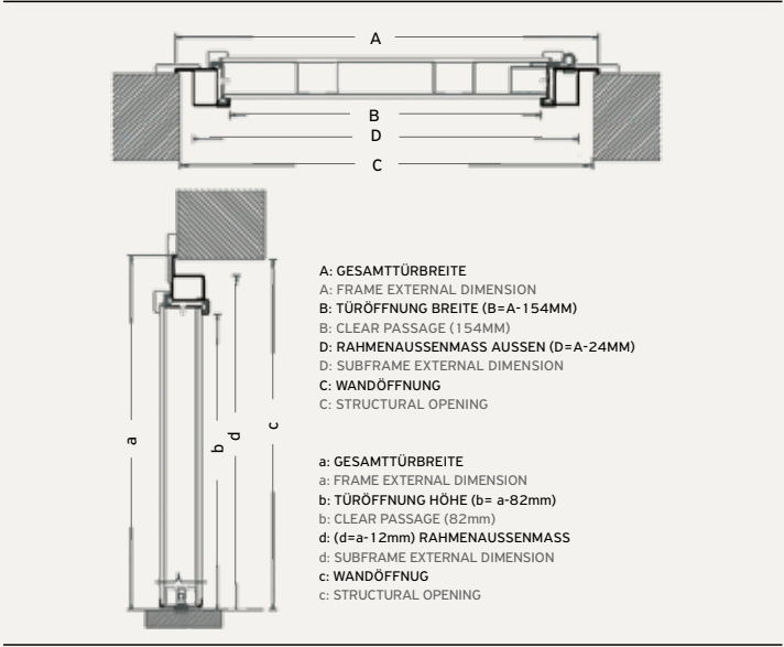
ANSICHT MIT ZARGE AUS ALUMINIUM POSITION VIEW WITH ALUMINIUM DECORATIVES
